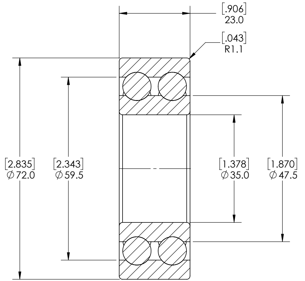
SECTION A-A
